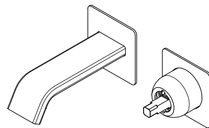
Vista ISO
