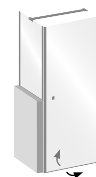
MOD. SINISTRO CON MANIGLIA A SINISTRA LATO FISSO SOPRAMURETTO A SINISTRA
